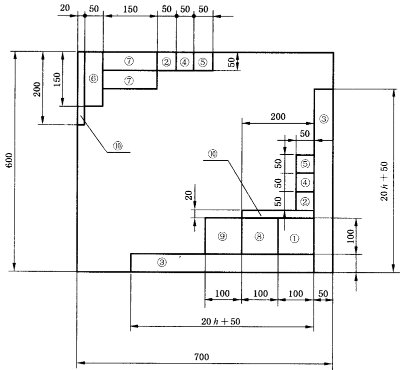
图 2 在 1、3、5 号试样上制取部分物理力学性能试件示意图 表 5 浸渍胶膜纸饰面人造板理化性能试件
