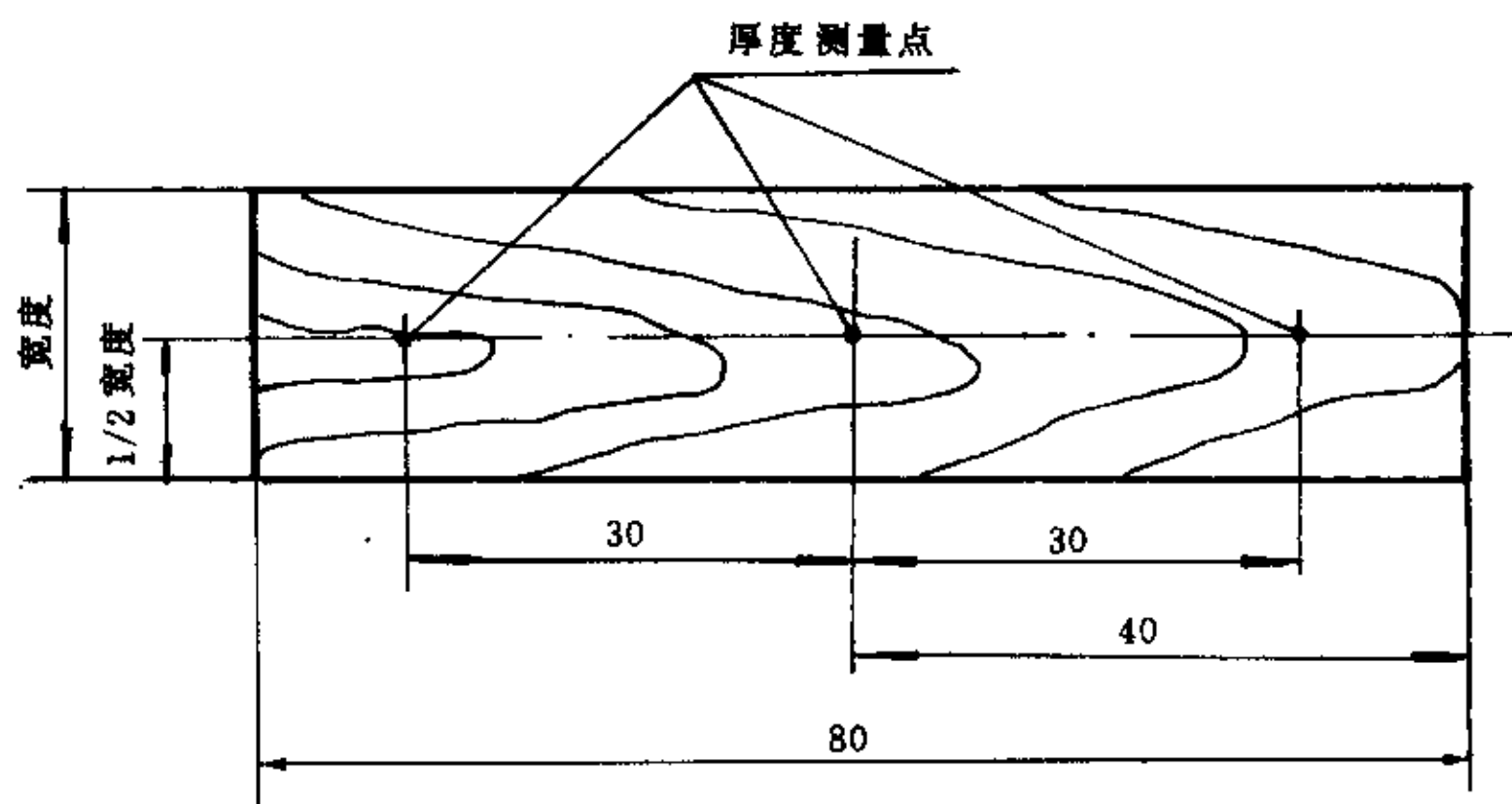
图 4 厚度测量
