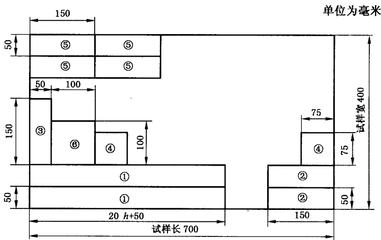
图 2 试件的配置示意图
